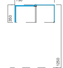
OPÇÃO: VDA UV vidro direito alto high flat frontal glass vitrage droit haut vidrio reto alto
