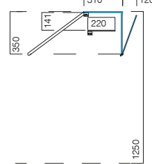
OPÇÃO: VDA vidro direito alto c/ prateleira high flat glass w/ shelf vitrage droit haut avec étagère vidrio reto alto c/ estante
