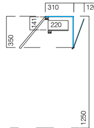
OPÇÃO: VDA vidro direito alto c/ prateleira high flat glass w/ shelf vitrage droit haut avec étagère vidrio reto alto c/ estante
