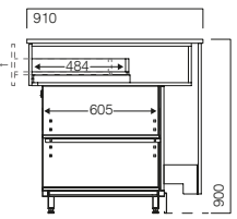
CX1N MIN B caixa support counter caisse caja
