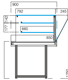
VMIN TV P torre de vidro glass tower tour de verre torre de cristal
