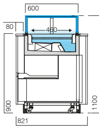
IMINSVS - VDB UV 3M2 ventilada ventilée ventilada
