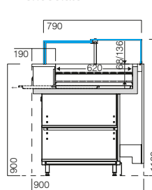
VMINPD B - VDB UV padaria bakery boulangerie panadería
