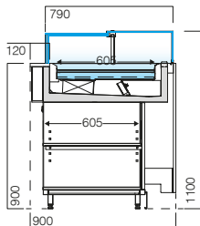
VMINVS - VDB UV 3M2 ventilada superior upper ventilated ventilée supérieure ventilada superior
