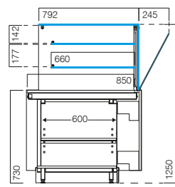
VMIN TV B torre de vidro glass tower tour de verre torre de cristal
