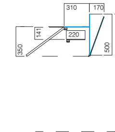
OPÇÃO: VDAP vidro direito alto c/ prateleira e pala higiénica high flat glass w/ shelf and sneeze guard vitrage droit haut avec étagère et para haleine vidrio reto alto c/ estante y anti-estornudos
