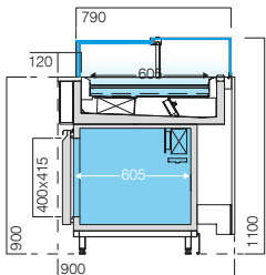
VMINVT - VDB UV 3M2 ventilada total total ventilated ventilée total ventilada total
