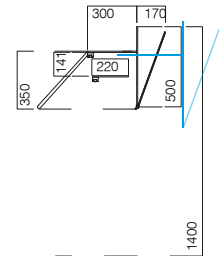
OPÇÃO: VDA P v.d.a. c/ prateleira e pala higiénica h.f.g. w/ shelf and sneeze guard v.d.h. avec étagère et para haleine v.r.a. c/ estante y anti-estornudos
