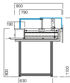
VMINPD P - VDB UV padaria bakery boulangerie panadería
