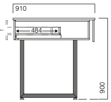
CX1N MIN P caixa support counter caisse caja
