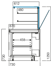
VMINSTV torre de vidro glass tower tour de verre torre de cristal
